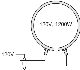
120 VOLT CONFIGURATION 1200 WATT
